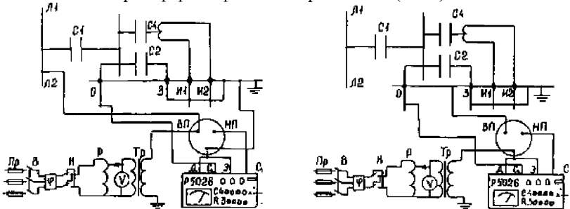
Рисунок Г.1 Схемы измерений тангенса угла диэлектрических потерь трансформаторов тока серии ТФЗМ (ТФН)
