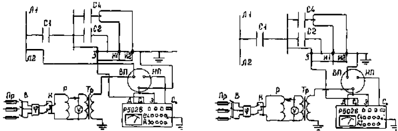
а) основной изоляции по нормальной схеме
