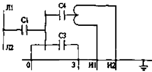
а) серия ТФМ (ТРН), типа ТФМ-330
