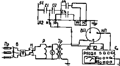
Рисунок Г.3 – Схемы измерений тангенса угла диэлектрических потерь трансформаторов тока серии ТФКН-330
